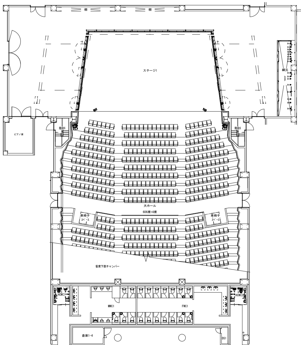
1階平面図
